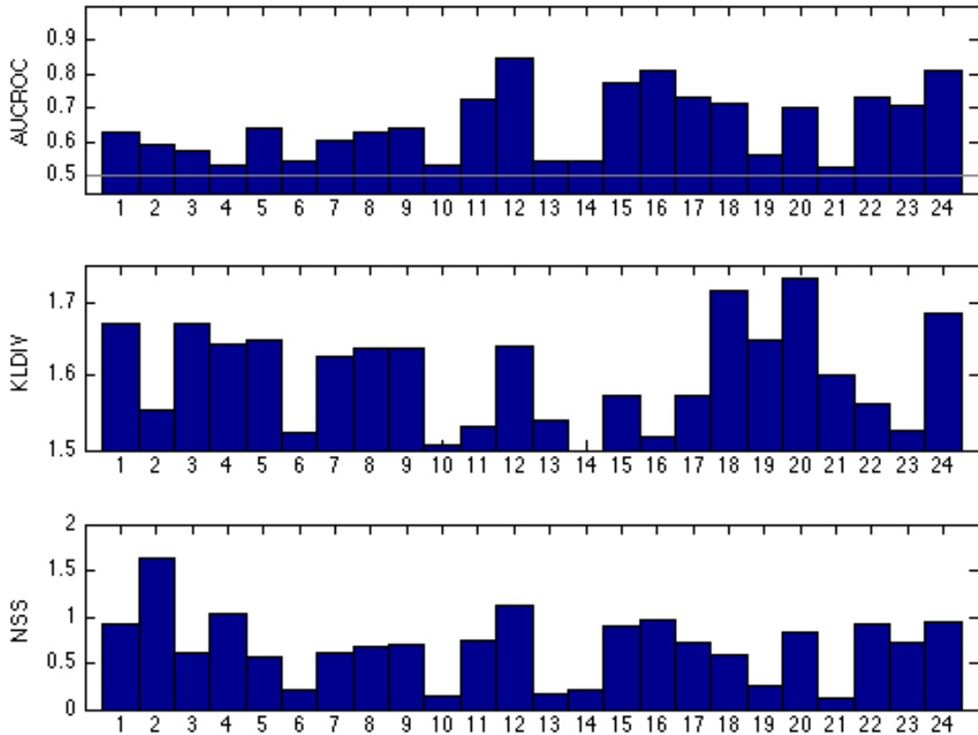
Obr. 4.6: Vizualizácia všetkých testovaných metrick pre dataset ASCMN[24] pre jednotlivé videá
